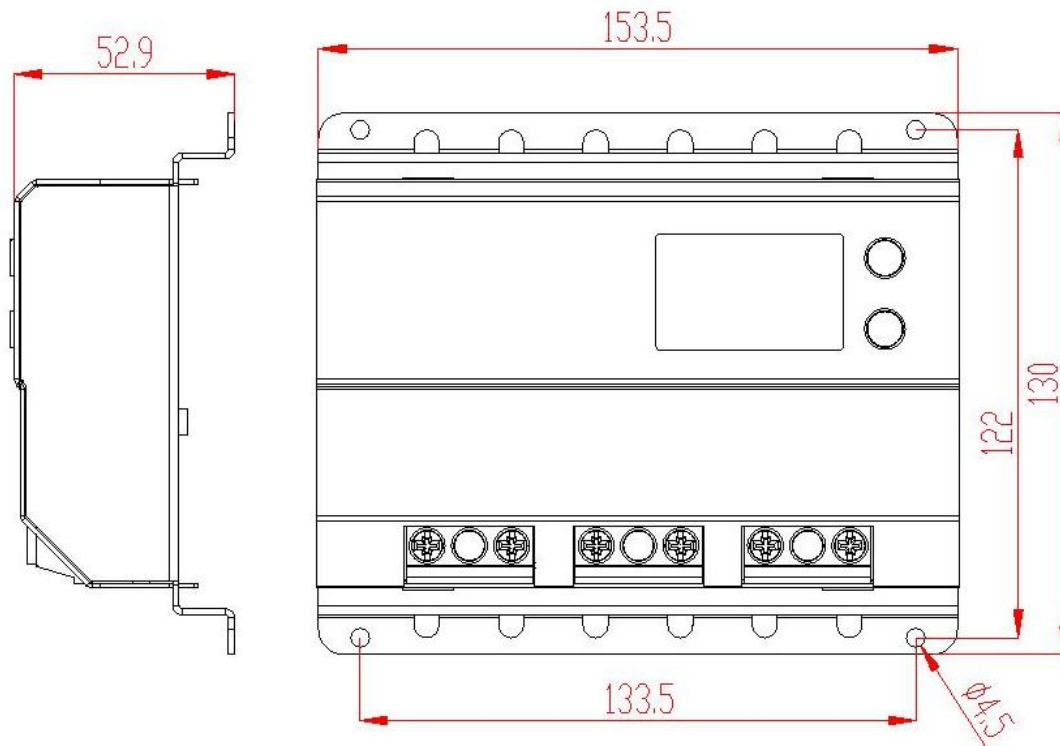
Fig. 8 Dimensioni
